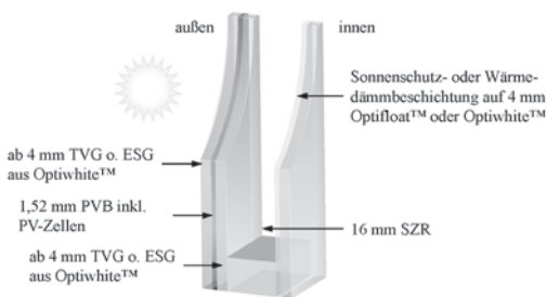
Zweischeiben-Isolierglas mit Pilkington Sunplus™ BIPV
