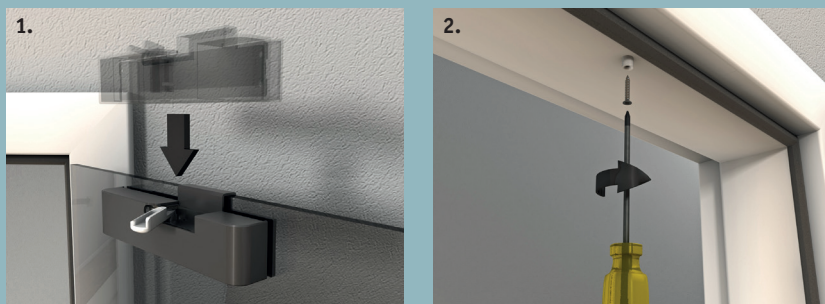
Einfache Montage: 1.) vetroMatic wird auf die Tür aufgeschoben 2.) An der Zarge ist lediglich ein kleiner Zapfen zu verschrauben
